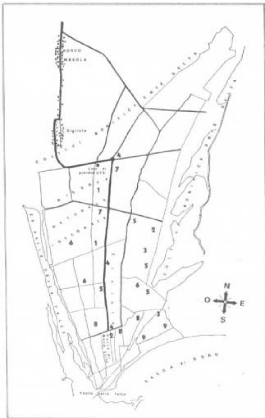
Attuale situazione topografica del «boscone» della Mesola (da Minerbi e altri, ridisegnato e modificato). I numeri indicano le stazioni di raccolta (vedi testo).
